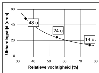
Diagram 1: Uithardingstijd voor 500 µm lijmlaag bij 20°C
