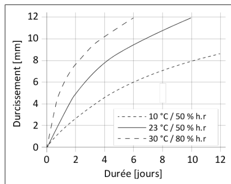
Diagramme 1 : Vitesse de polymérisation du SikaTack® Panel
