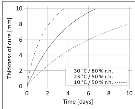
Grafiek 1: Doorhardingssnelheid Sikaflex®-263
