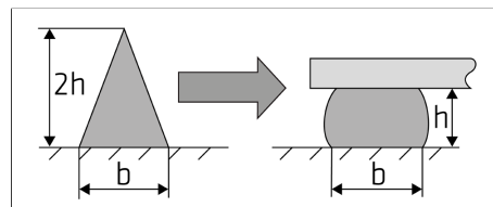
Figuur 1: Aanbevolen lijmrups configuratie
