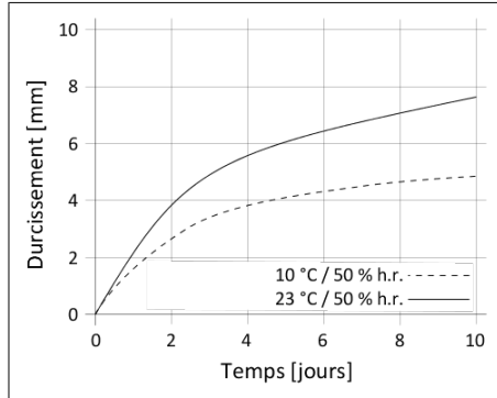
Diagramme 1: Vitesse de polymérisation du Sikaflex®-521 UV
