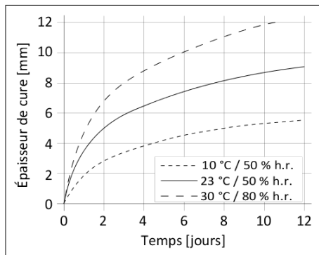
Diagramme 1: temps de polymérisation du Sikaflex®-260 N
