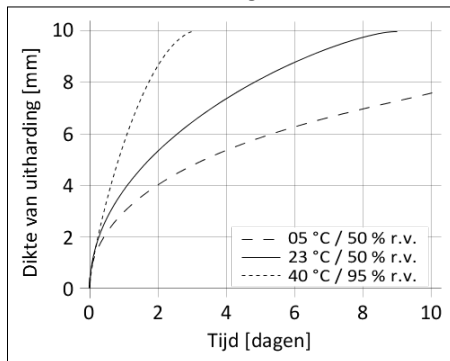
Schema1: Uithardingsnelheid Sikasil® WS-200
