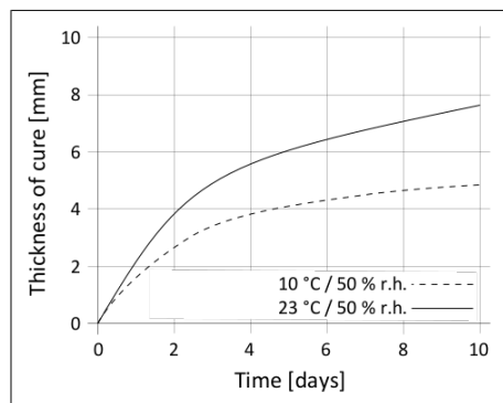
Diagram 1: Uithardingsssnelheid Sikaflex®-529 Evolution
